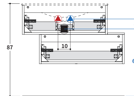
VISTA RETRO Rear view / Vue arrière / Rückansicht
