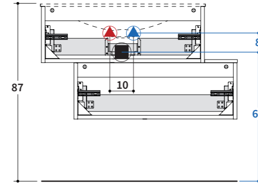
VISTA RETRO Rear view / Vue arrière / Rückansicht
