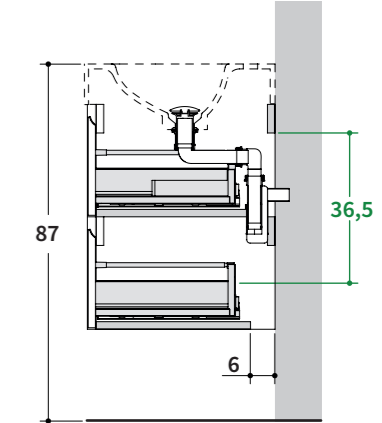
VISTA IN SEZIONE Lateral view / Vue latérale / Seitenansicht
